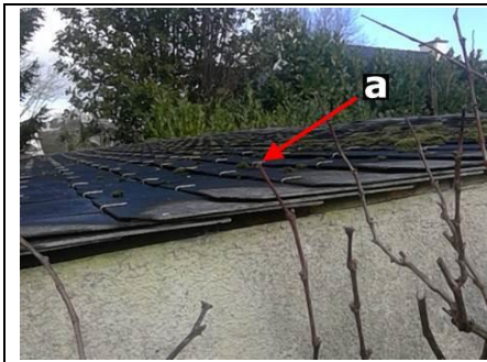
Photo n° PhA001 Localisation : Abris de jardin Ouvrage : Toitures Partie d'ouvrage : Ardoises (composites) Description : Ardoises (composites)
